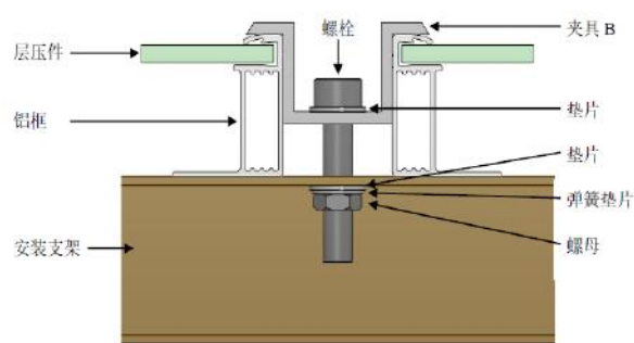
中间压块
